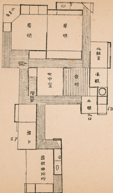
階下平面圖
