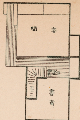
階上平面圖
