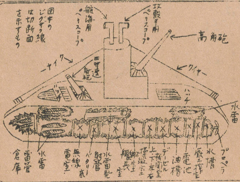
英国が捕獲せし独逸Uボートその神経系統解剖略図
